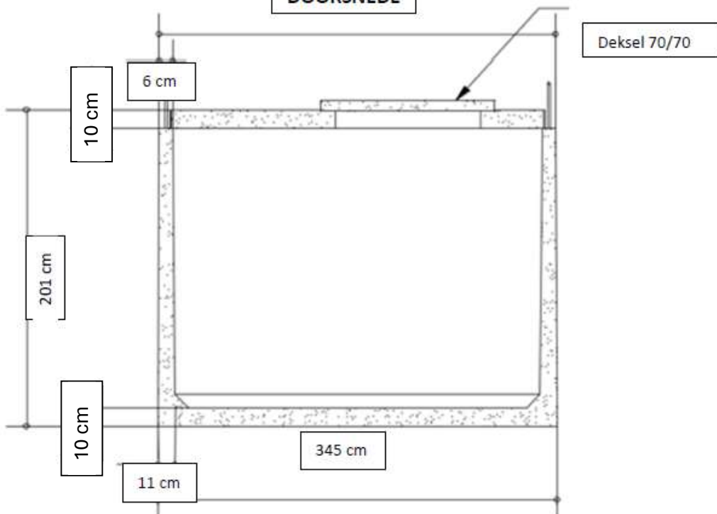
DOORSNEDE
